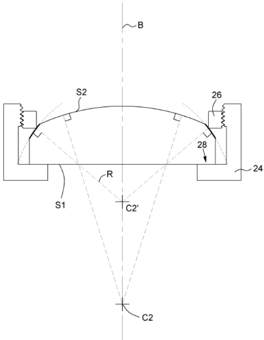
FIG. 11C
