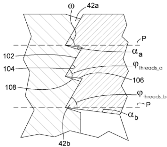
FIG. 24B
