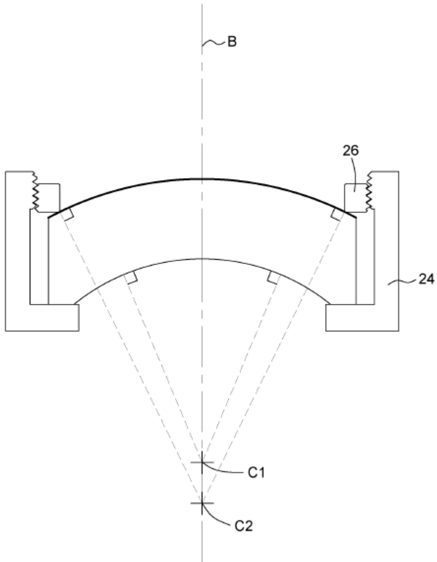
FIG. 10B
