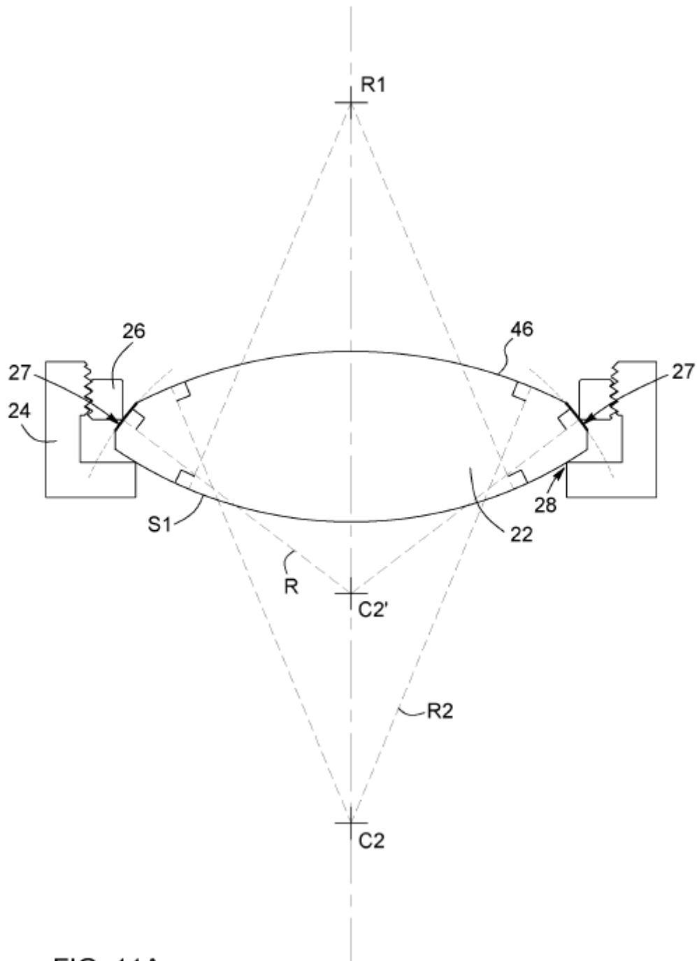
FIG. 11A
