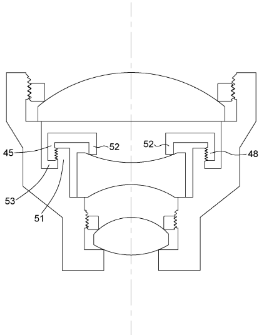
FIG. 14A
