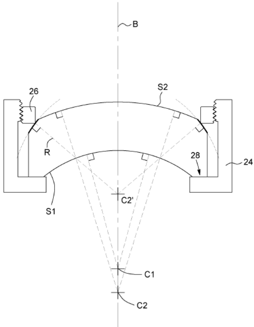
FIG. 11B
